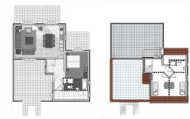
Begane grond
